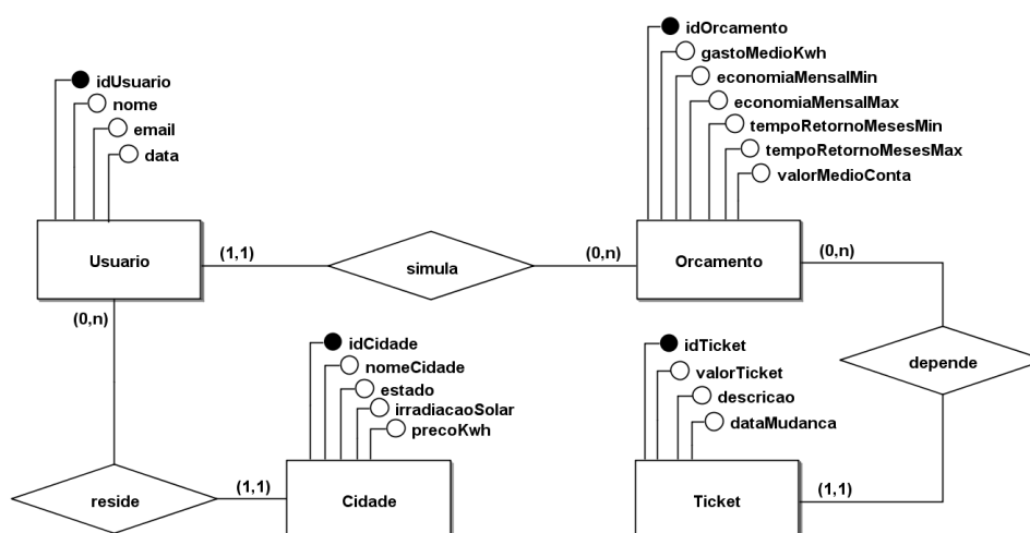
Figura 2 – Diagrama Entidade-Relacionamento do SolarEasy
